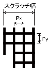
格子形のキズ間隔 (mm) 周方向 : P_x=0.4 径方向 : P_y=0.4
