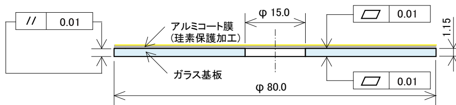
SCD-4142の寸法図
