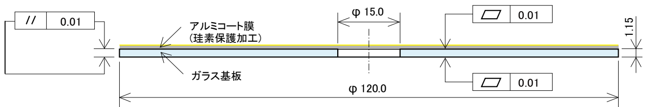
SCD-4143の寸法図
