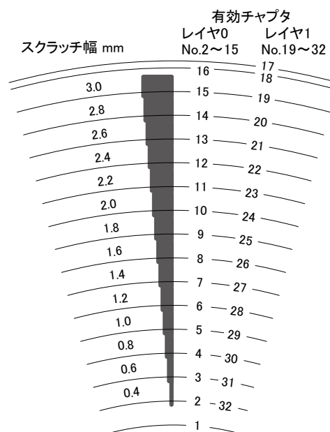
スクラッチとチャプタの位置関係
