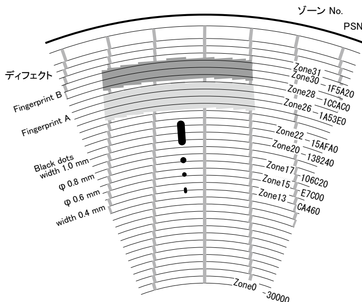
ディフェクトとPSNアドレス、ゾーンの位置関係
