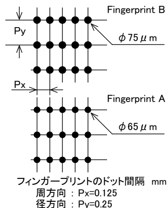
イメージ図③ フィンガープリントの詳細図
